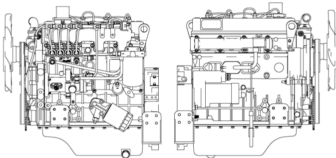
Общий вид дизельного двигателя 4DW91-50GBG3U
