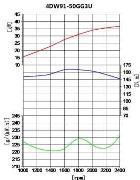
Мощностные характеристики двигателя от оборотов
