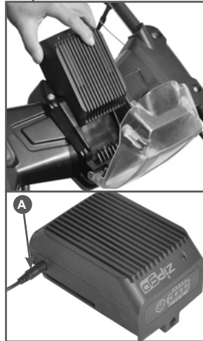
Рис. 19 Зарядка аккумулятора
