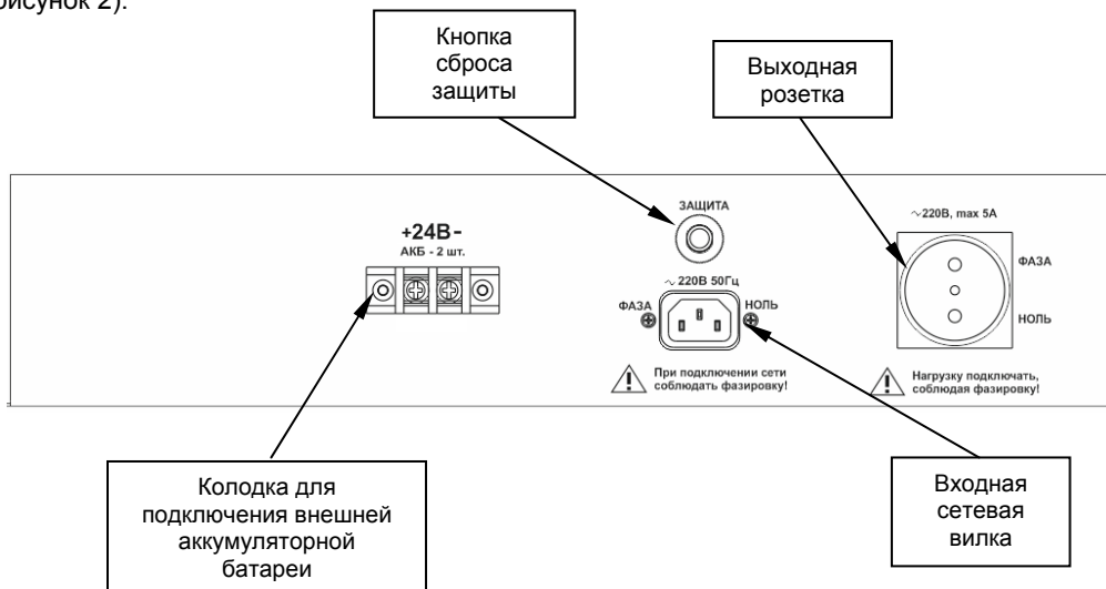
Рисунок 2. Расположение разъемов для подключения.
