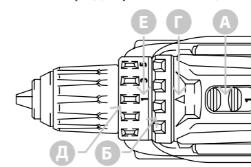
Рисунок 2.3.4. Работа в режиме шуруповерта
