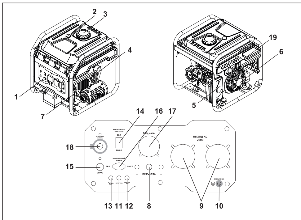
Рис. 9 Общий вид модели BR5000iOL
