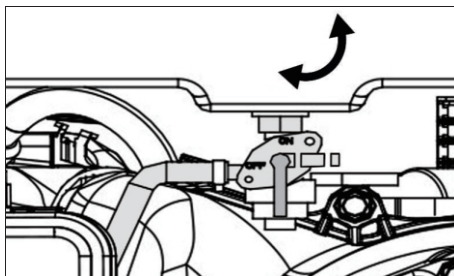
Рис. 22 Топливный кран
