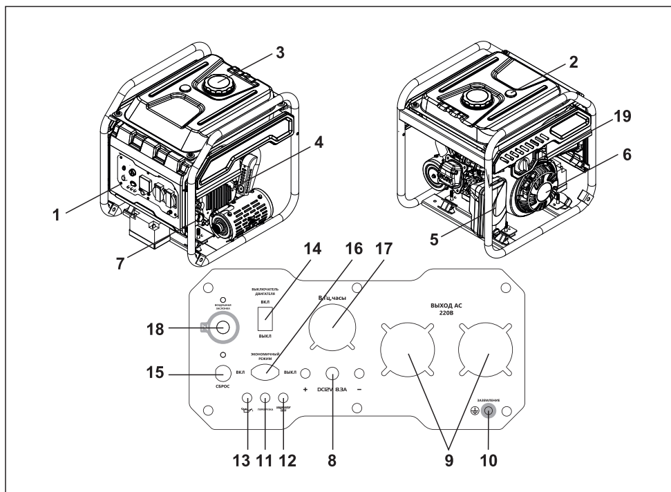
Рис. 14 Общий вид модели BR7500iOEL
