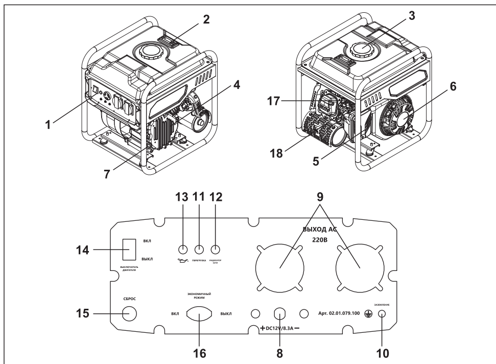
Рис. 12 Общий вид модели BR7500iO
