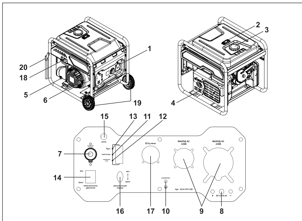
Рис. 15 Общий вид модели BR8500iOM
