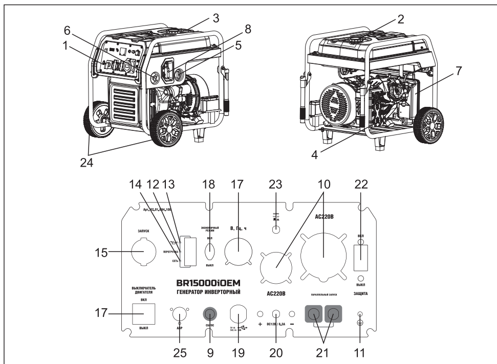
Рис. 17 Общий вид модели BR15000iOEM
