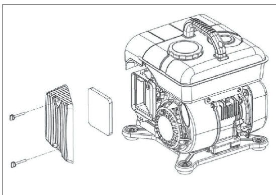
Рис. 29 Воздушный фильтр
