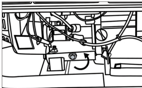
Рис. 26 Слив масла
