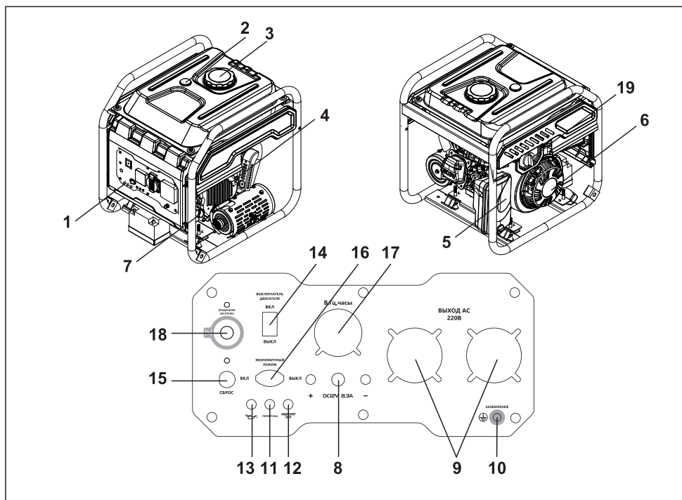
Рис. 13 Общий вид модели BR7500iOL
