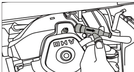
Рис. 27 Высоковольтный провод и свеча зажигания
