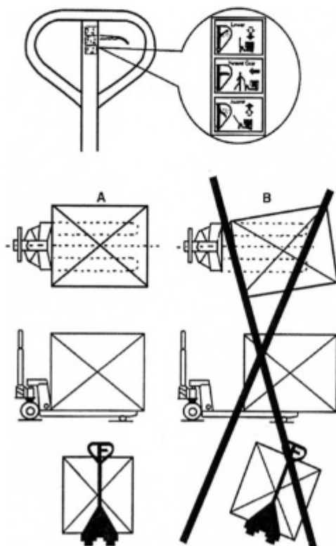
Рисунок 4. Расположение груза.
