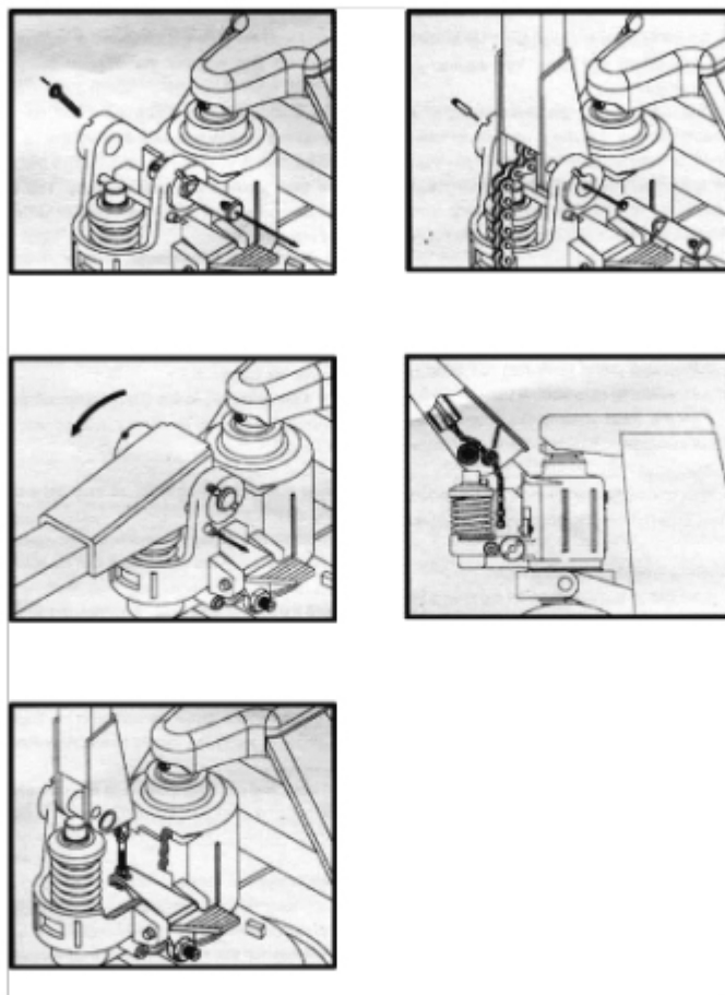
Рисунок 2. Установка ручки тележки.
