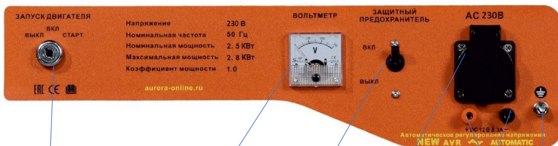
Замок зажигания Вольтметр Защитный предохранитель Выход 230В Заземление Выход DC 12В, 8.3А
