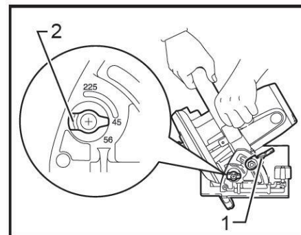
1. Фиксатор 2. Регулировочный винт
