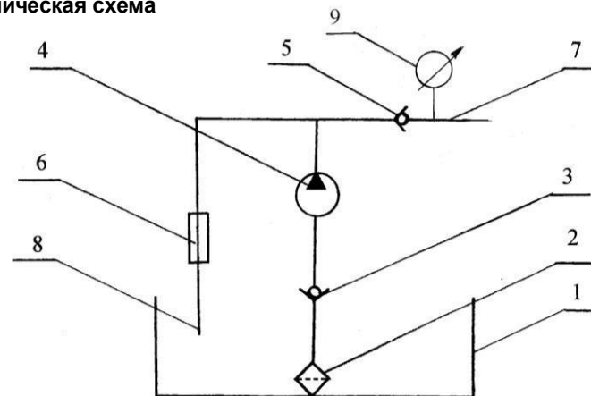
Рис. 1 Гидравлическая схема
