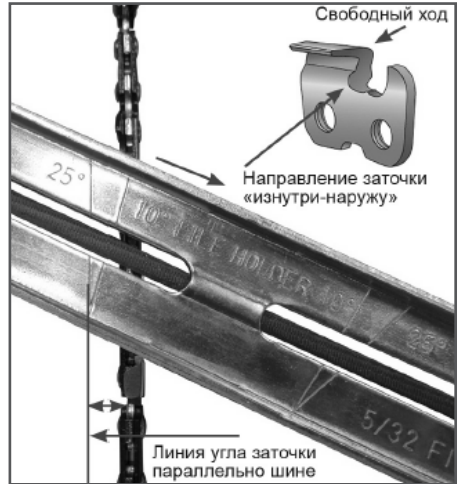
Рис. 28 Определение угла заточки
