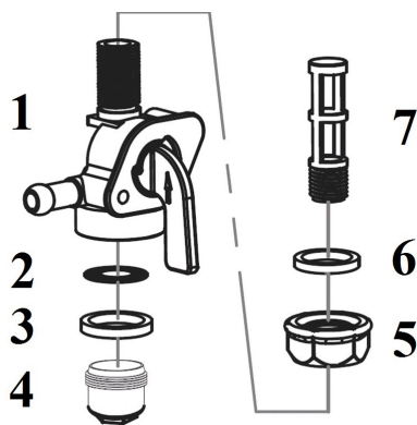
Рис. 19 Устройство топливного крана
