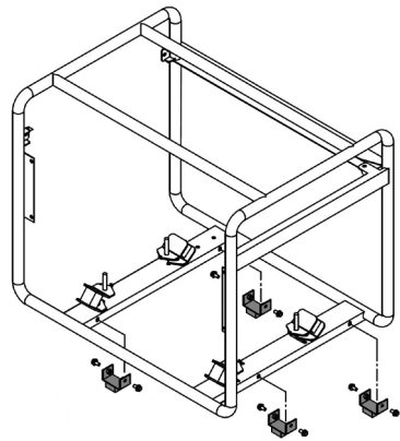
Рис. 4 Установка опор рамы
