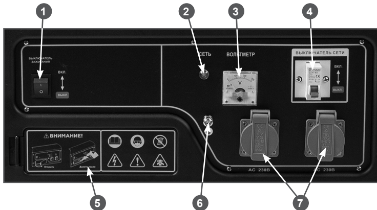
Рис. 3 Панель управления
