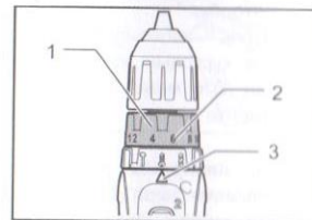
1. Регулировочное кольцо 2. Градуировка 3. Стрелка
