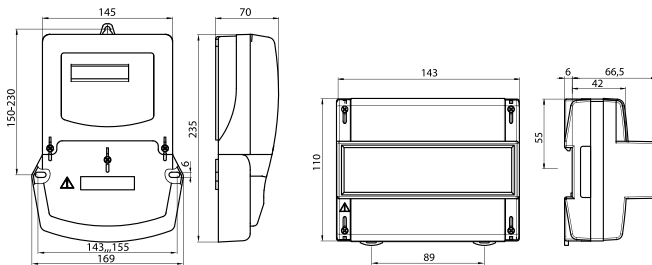
Рисунок А.3 — Тип корпуса ШЗЗ
