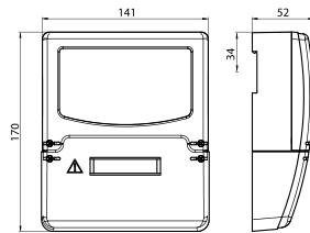
Рисунок А.1 — Тип корпуса P32
