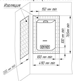
Рисунок 2. Установка аппарата на трудносгораемых стенах
