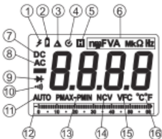
Рис. 3 Дисплей, вид 2
