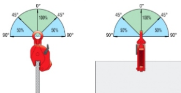
Рисунок 6. Рабочая нагрузка в соответствии с различными углами
