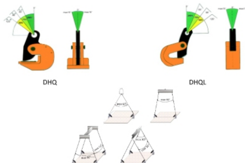
Рисунок 2. Рабочая нагрузка в соответствии с различными углами
