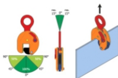
Рисунок 4. Рабочая нагрузка в соответствии с различными углами
