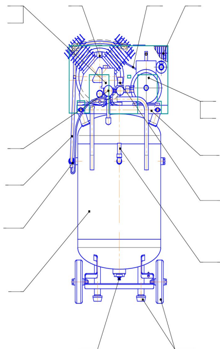
Рисунок 8 - Общий вид компрессоров СБ4/С-100.LB30В, СБ4/С-100.LB30АВ
