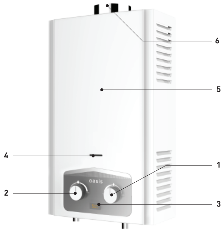
Рис. 1. Аппарат водонагревательный проточный газовый бытовой «OASIS» 1 - ручка водяного регулятора; 2 - ручка газового регулятора; 3 - цифровой дисплей с индикацией температуры и заряда батареи; 4 - окно смотровое; 5 - облицовка; 6 - дымоотводная труба.
