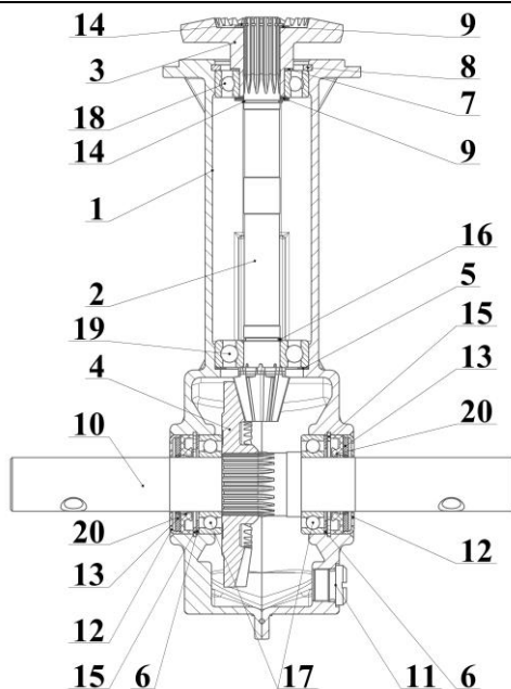
Рисунок 9 – Суппорт.
