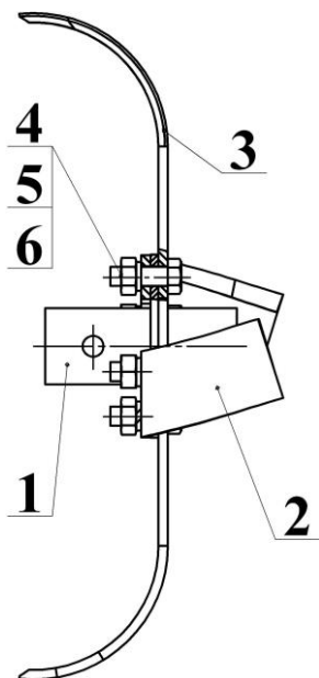
Рисунок 11а – Фреза КМБ1.001.030.4(-01).
