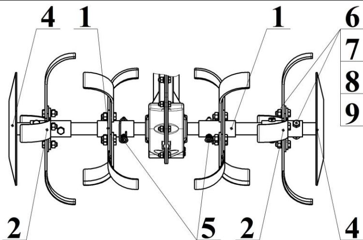
Рисунок 12б – Культиватор КМБ1.001.000.2-01.
