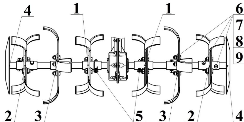
Рисунок 12г – Культиватор КМБ1.001.000.2-03.
