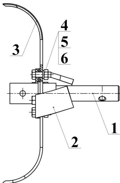
Рисунок 11б – Фреза КМБ1.001.010.7(-01).
