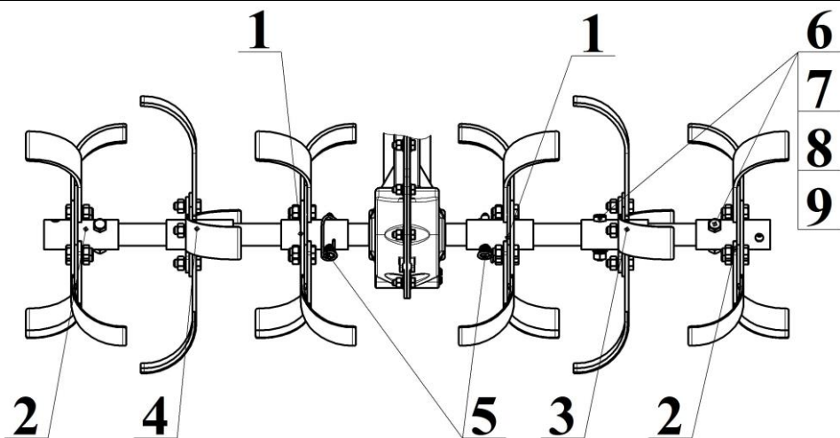
Рисунок 12в – Культиватор КМБ1.001.000.2-02.
