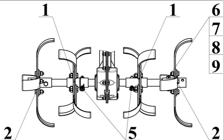
Рисунок 12а – Культиватор КМБ1.001.000.2.
