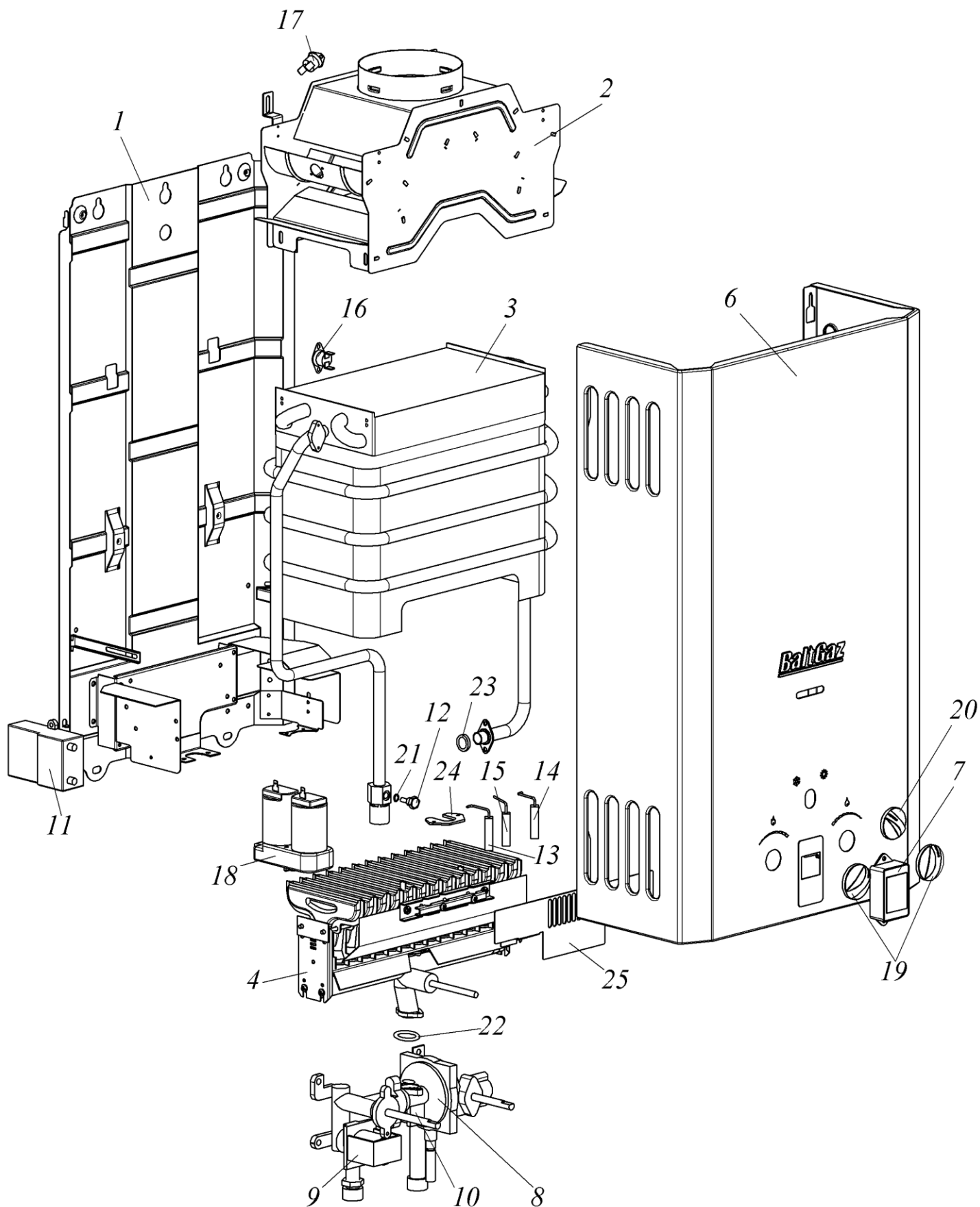
Рис. 11. Вид аппарата с разнесенными частями
