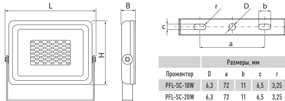
Рис. 1 Прожектор PFL-SC
