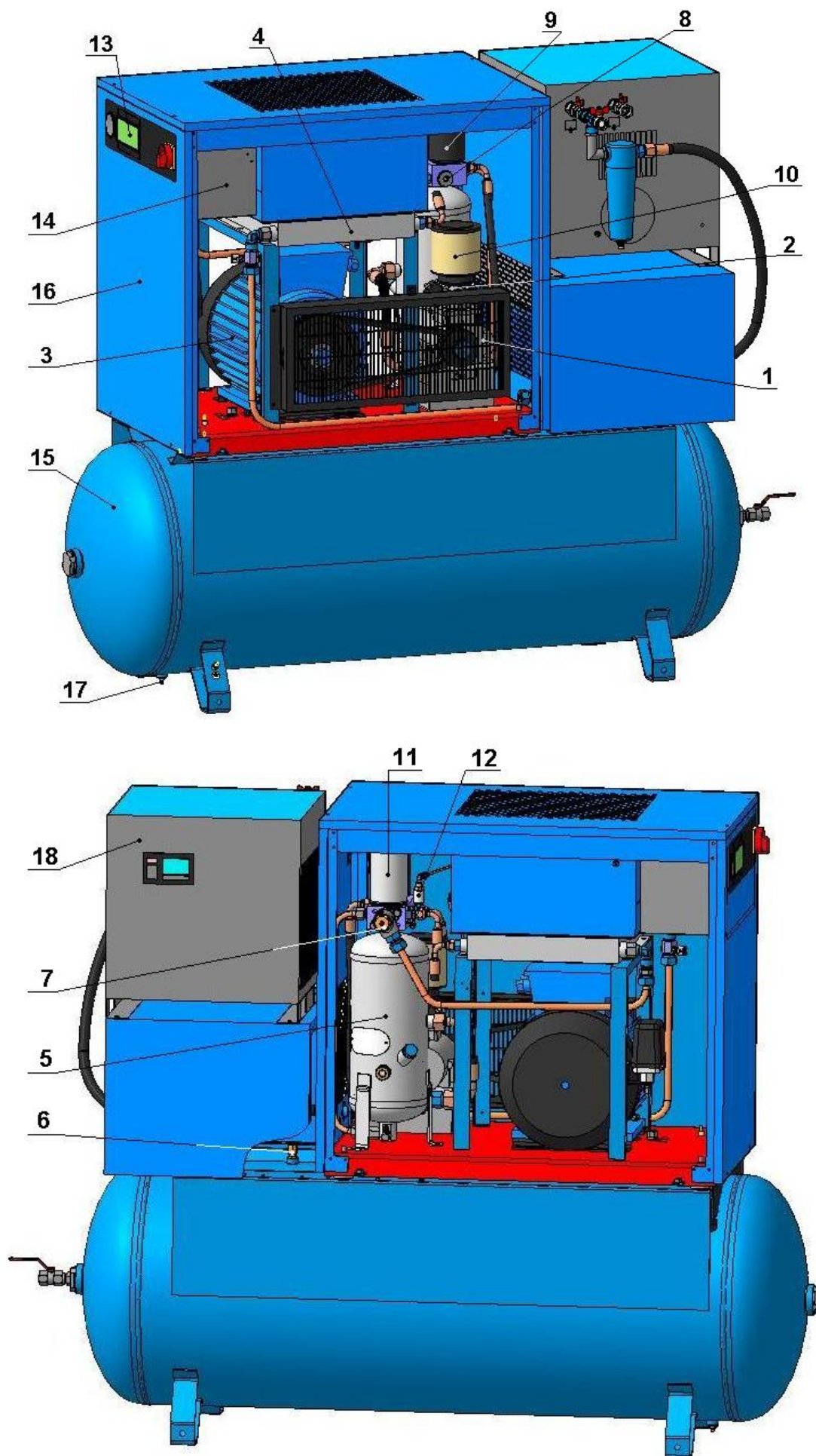
Рисунок 3 – Общий вид компрессорной установки BK20E-8(10, 15)-500Д
