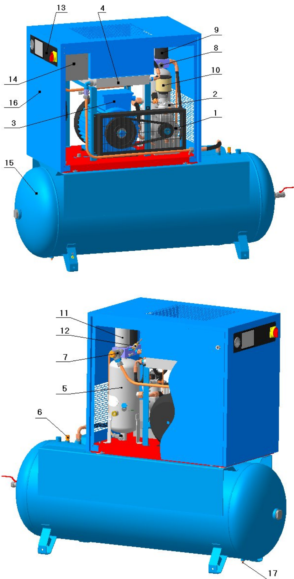
Рисунок 2 – Общий вид компрессорной установки BK20E-8(10, 15)-500
