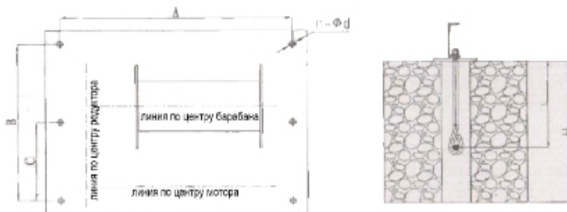
Рисунок 6. Разметка крепежных болтов.
