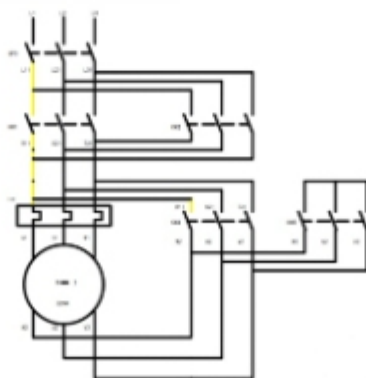
Рисунок 4.2 Электрическая схема лебедки ЛМ, г/п 10т.
