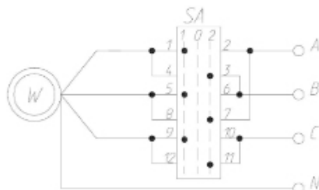
Рисунок 4.1 Электрическая схема лебедки ЛМ, г/п 0,5-5т.
