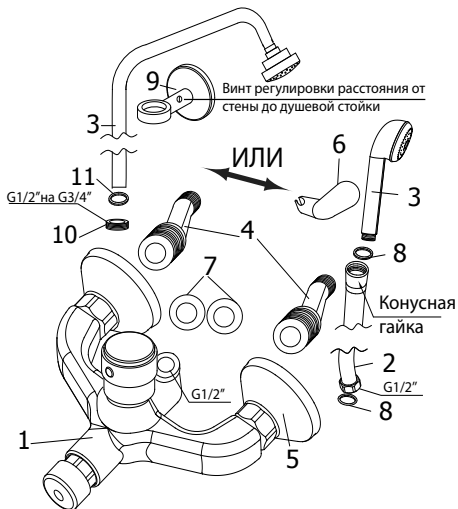
Установочная Схема №3.
