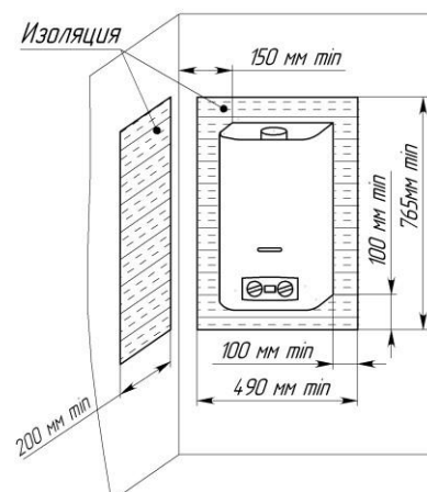
Рис. 5. Установка аппарата на труднодоступных стенках
