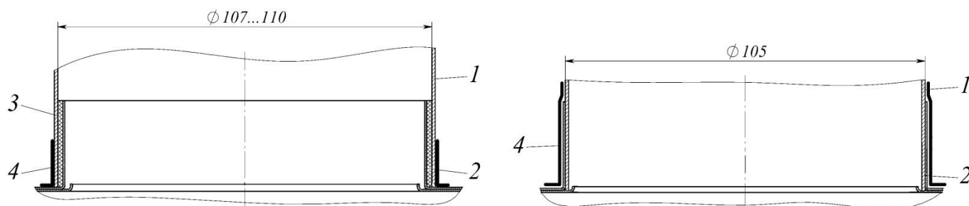
1 – газоотводящая труба; 3 – термостойкий уплотнитель 2 – патрубок газоотводящего устройства аппарата; 4 – скотч алюминиевый термостойкий
