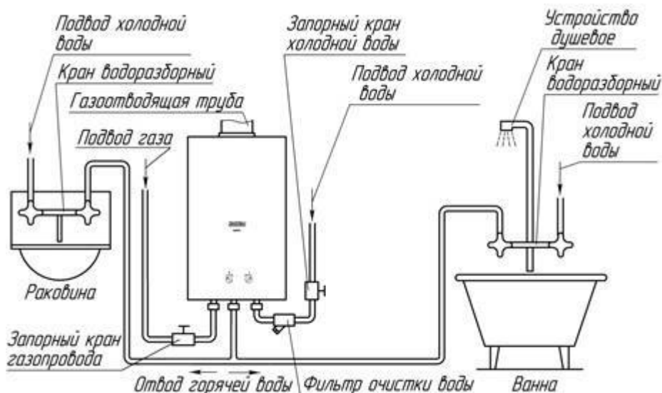
Рис. 6. Схема установки аппарата
