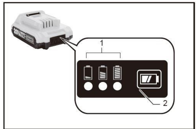
1. Индикаторные лампы 2. Кнопка проверки
