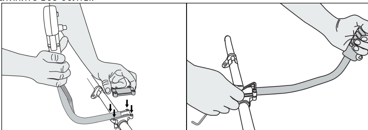
Рис. 3 Установка рукояток
