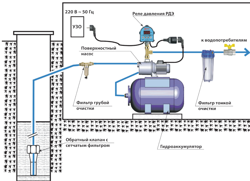
Схема 1. Подключение реле давления РДЭ "Extra "Акваконтроль" с поверхностным насосом
