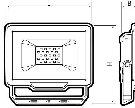
Рис. 1 Прожектор PFL-C3
