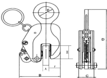
Рисунок 3. Размеры захвата
