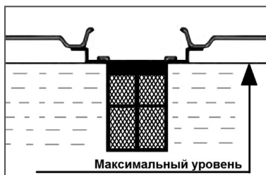
Рис. 10 Максимальный уровень топлива в топливном баке
